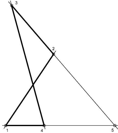
selbstüberschneidendes Viereck (Antiparallelogramm)
